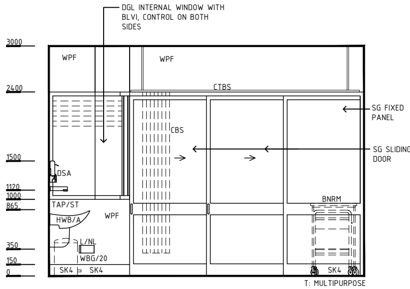
ELEVATION 3
