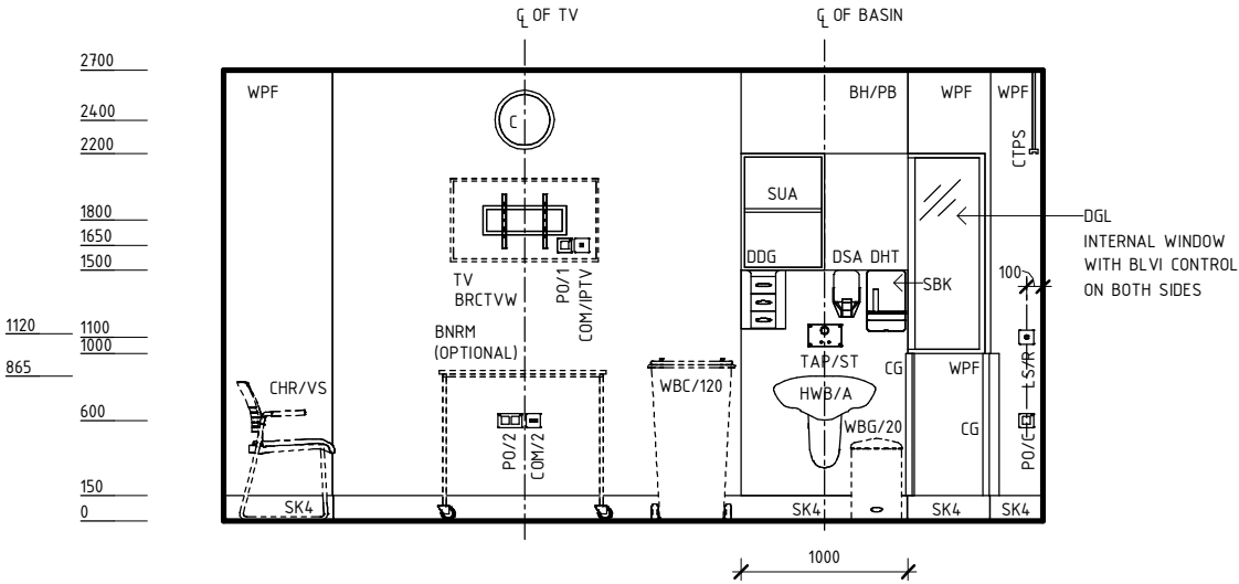
ELEVATION 2
