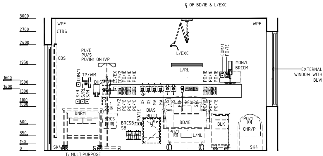
ELEVATION 4
