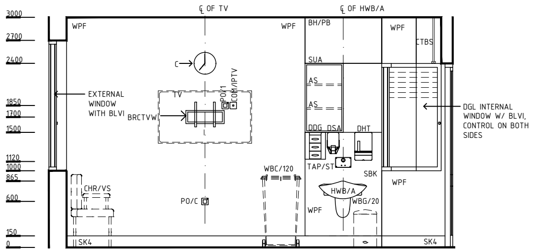
ELEVATION 2
