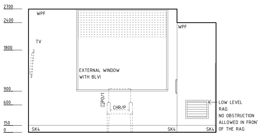
ELEVATION 1
