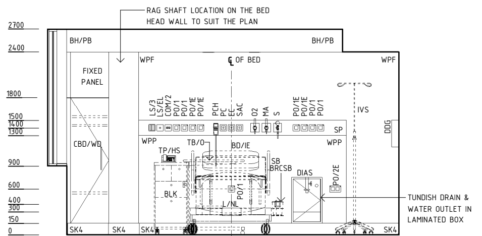
ELEVATION 2
