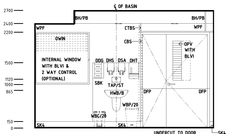
ELEVATION 3
