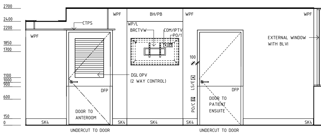
ELEVATION 4
