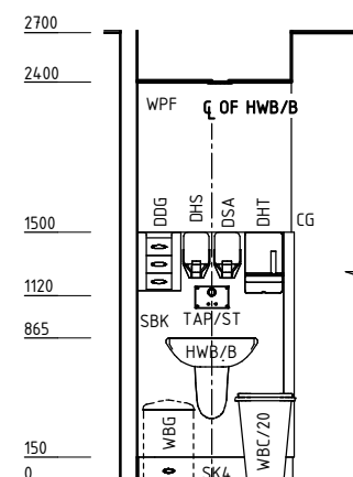
ELEVATION 6
