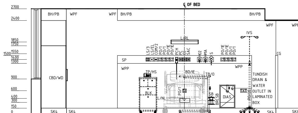
ELEVATION 2
