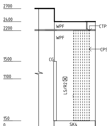
ELEVATION 5
