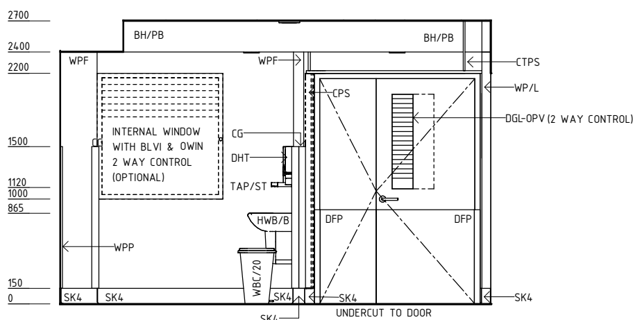
ELEVATION 3
