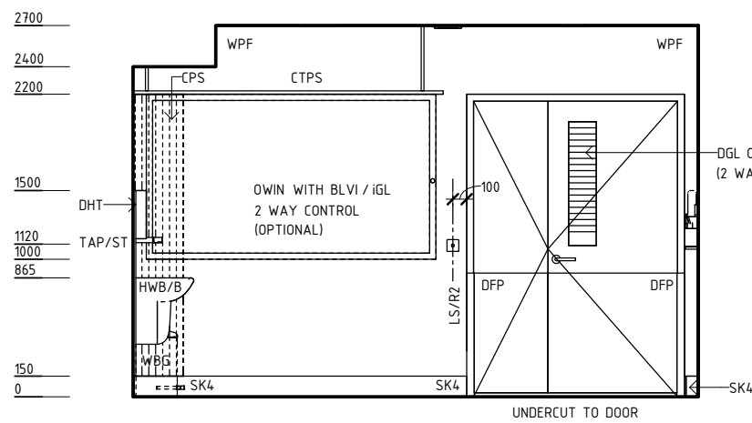
ELEVATION 3
