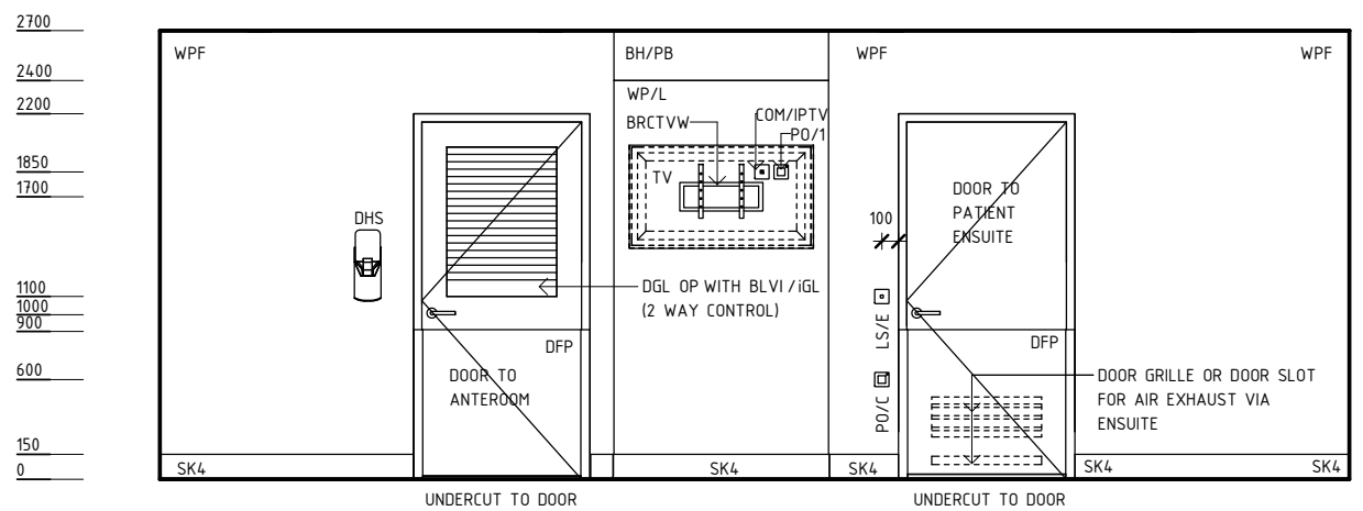
ELEVATION 4
