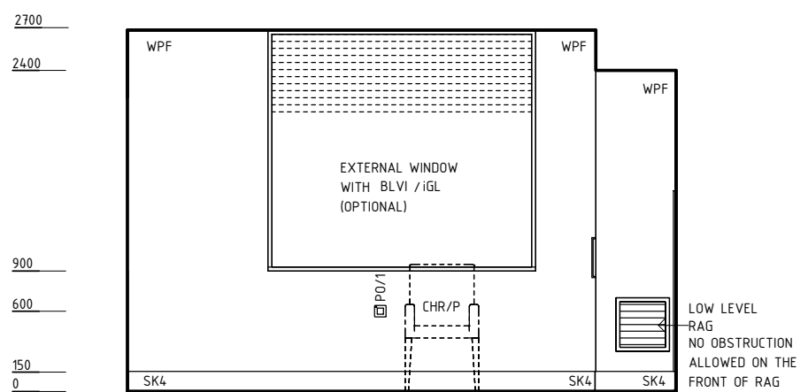
ELEVATION 1
