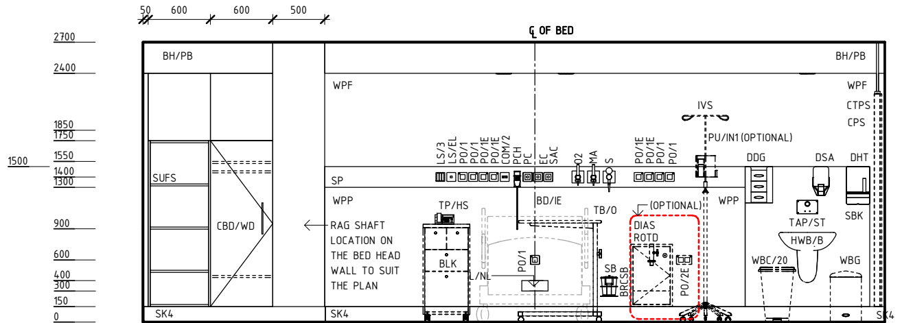
ELEVATION 2
