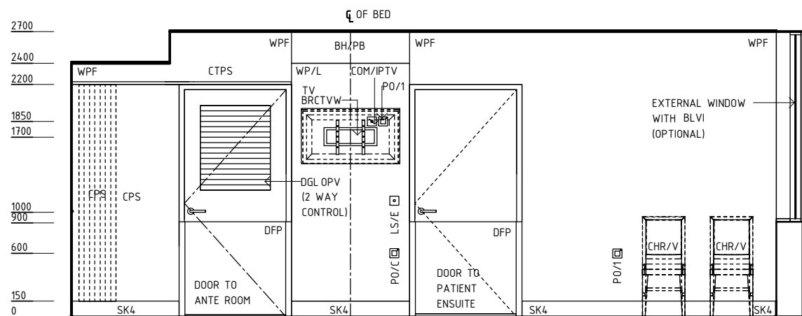
ELEVATION 4
