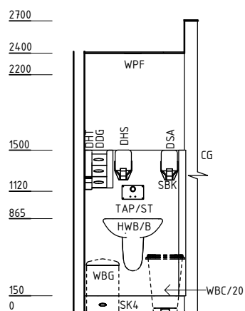
ELEVATION 6
