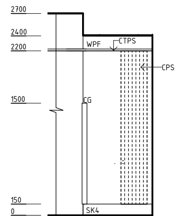
ELEVATION 5
