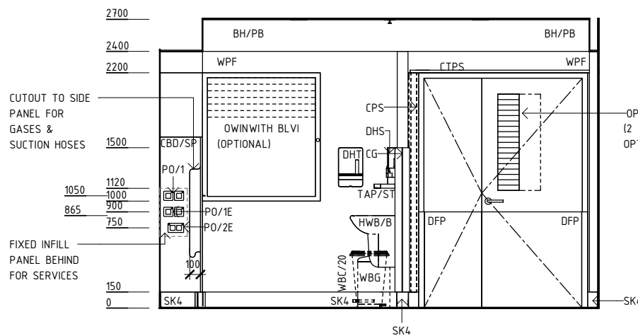
ELEVATION 3
