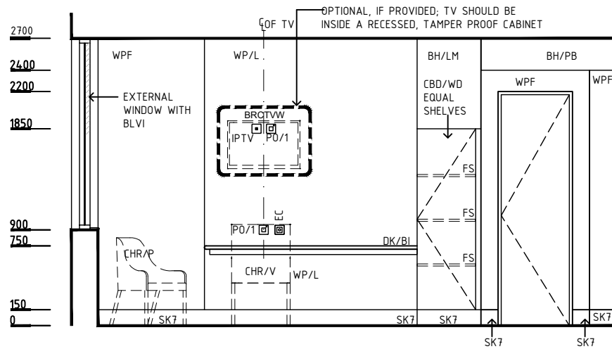
ELEVATION 2
