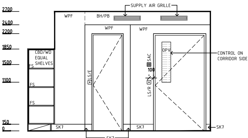
ELEVATION 3
