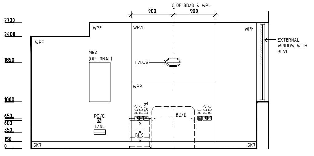
ELEVATION 4
