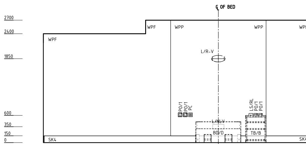
ELEVATION 4
