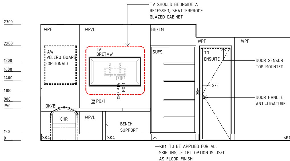
ELEVATION 2
