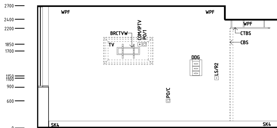
ELEVATION 2
