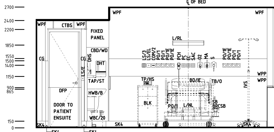
ELEVATION 4
