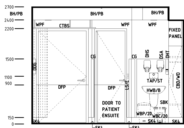
ELEVATION 3
