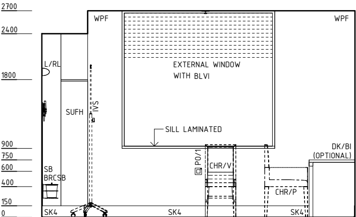
ELEVATION 1
