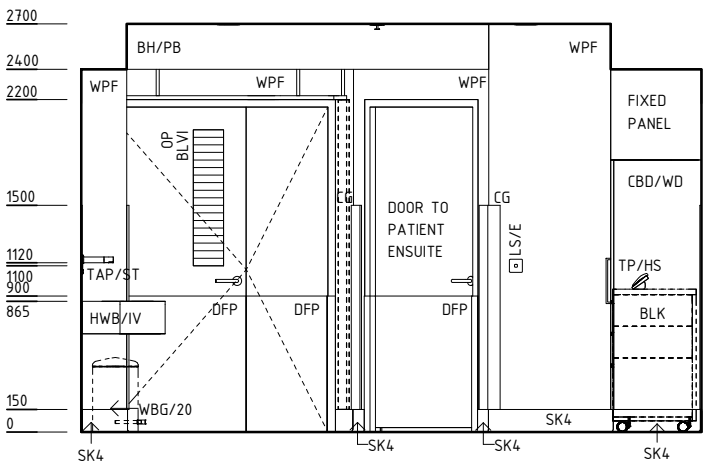
ELEVATION 3
