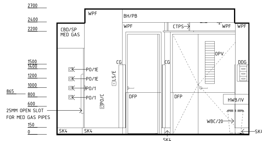
ELEVATION 3
