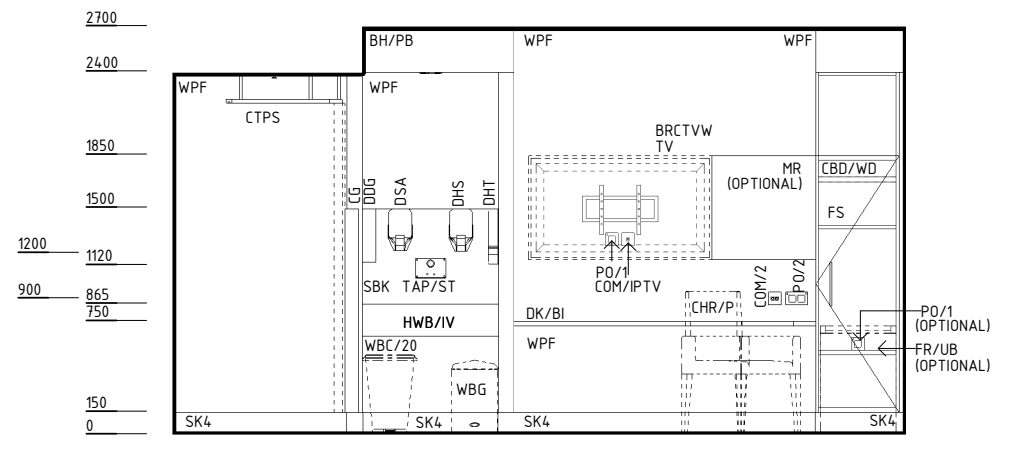
ELEVATION 4
