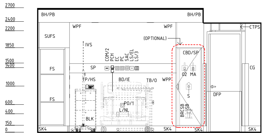
ELEVATION 2
