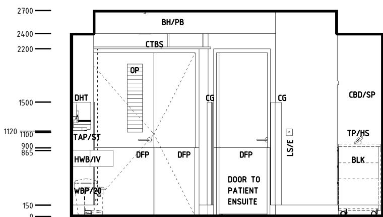
ELEVATION 3
