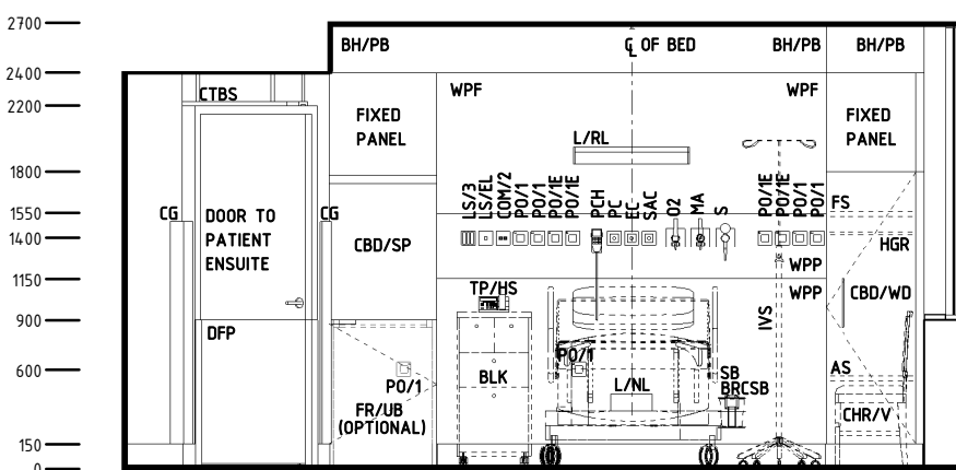
ELEVATION 4
