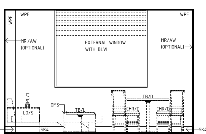
ELEVATION 5
