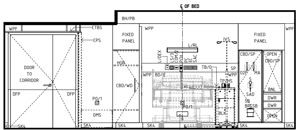
ELEVATION 3
