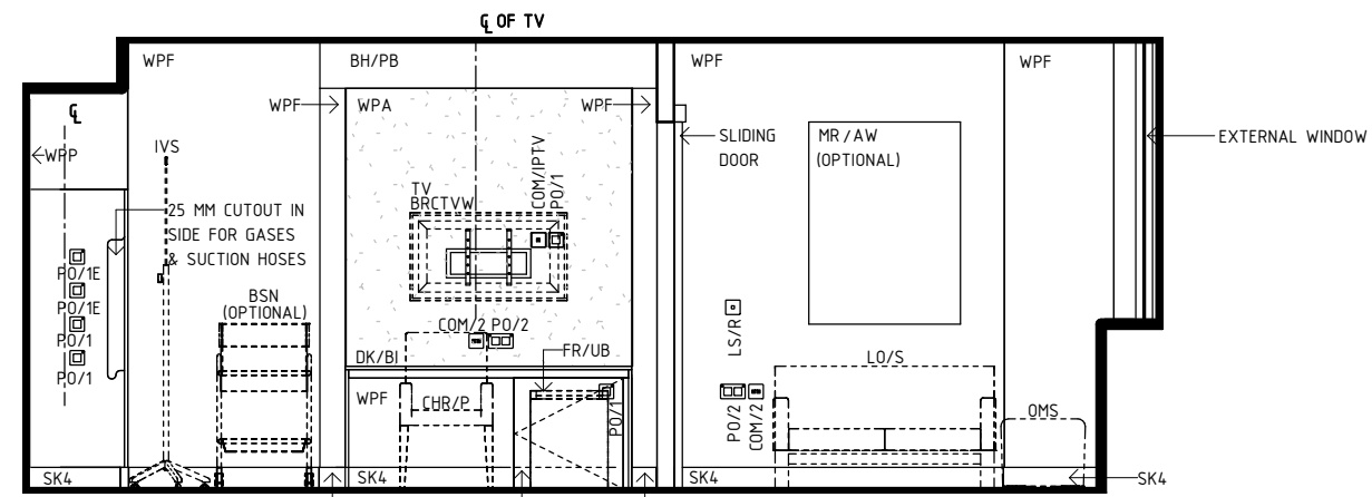
ELEVATION 4
