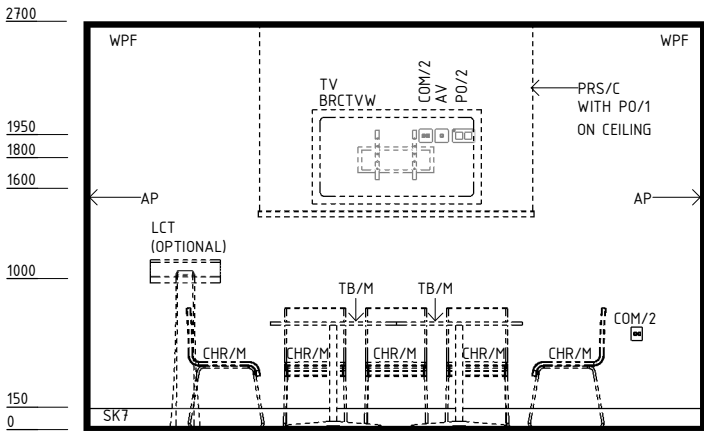
ELEVATION 1
