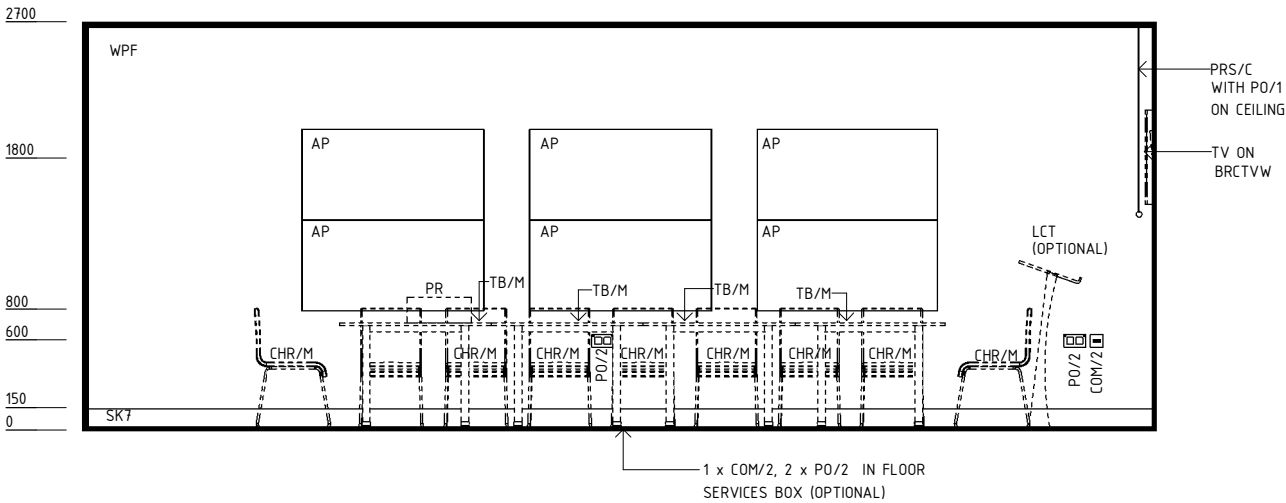
ELEVATION 4
