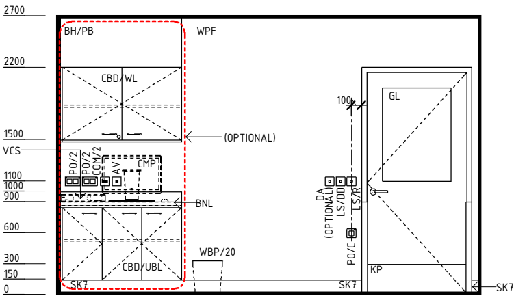
ELEVATION 3
