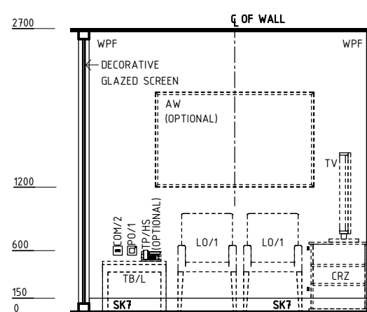
ELEVATION 3
