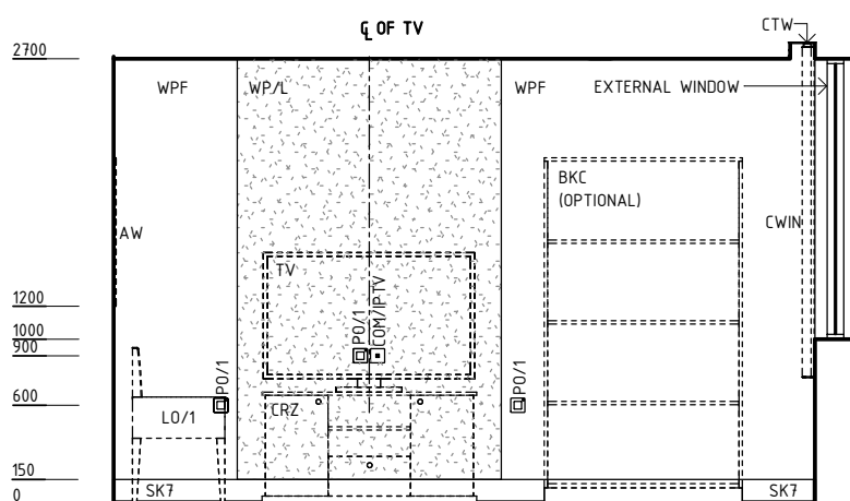
ELEVATION 4
