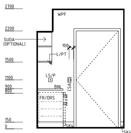
ELEVATION 1
