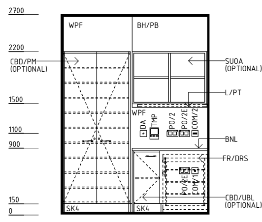
ELEVATION 3
