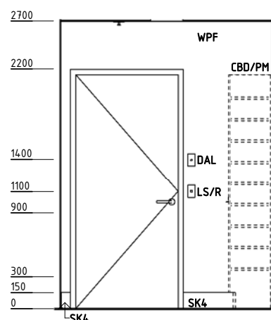
ELEVATION 2
