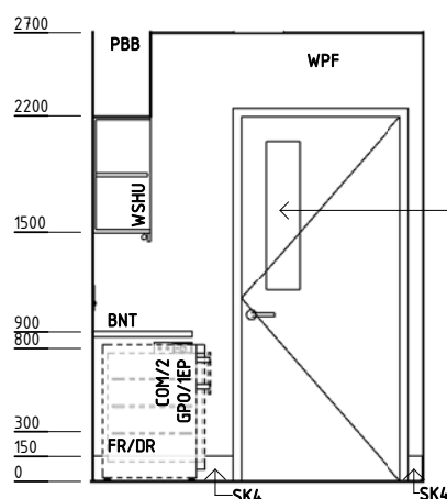
ELEVATION 1
