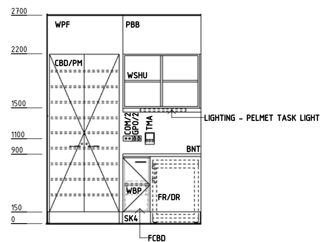
ELEVATION 3
