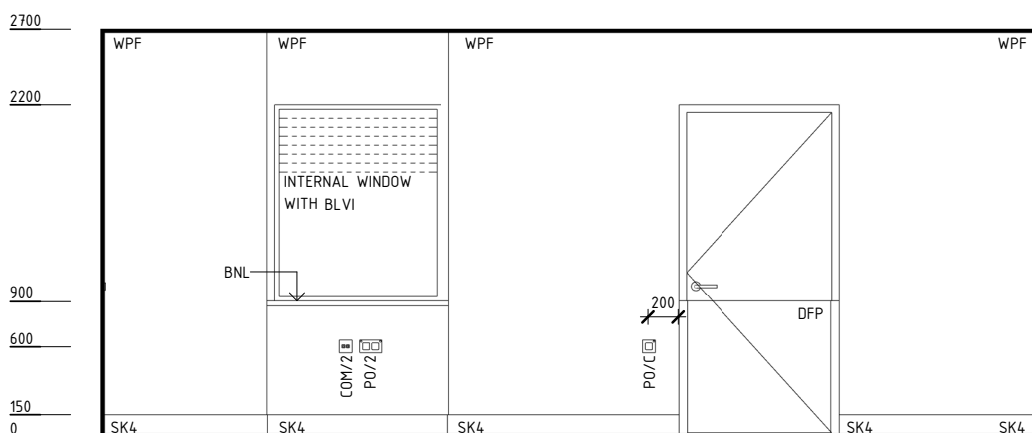
ELEVATION 3
