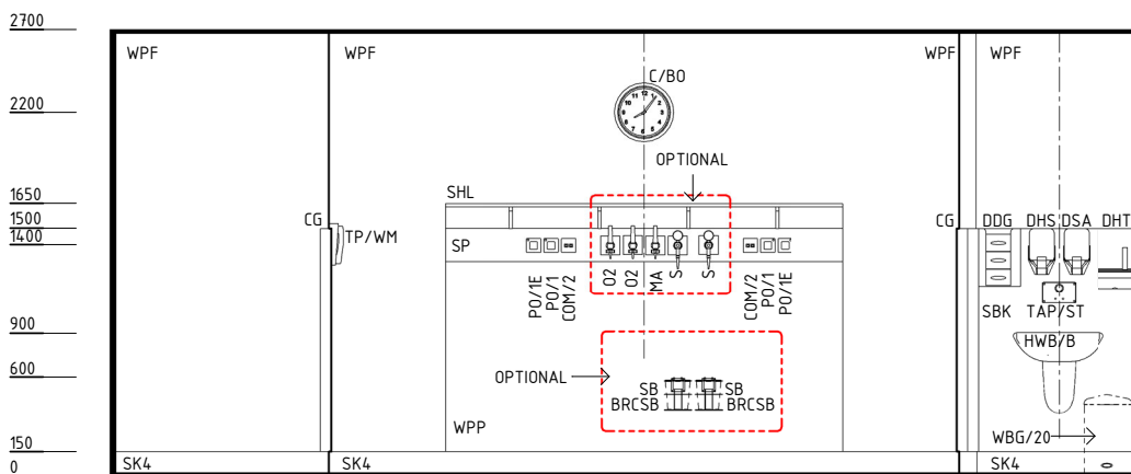
ELEVATION 1
