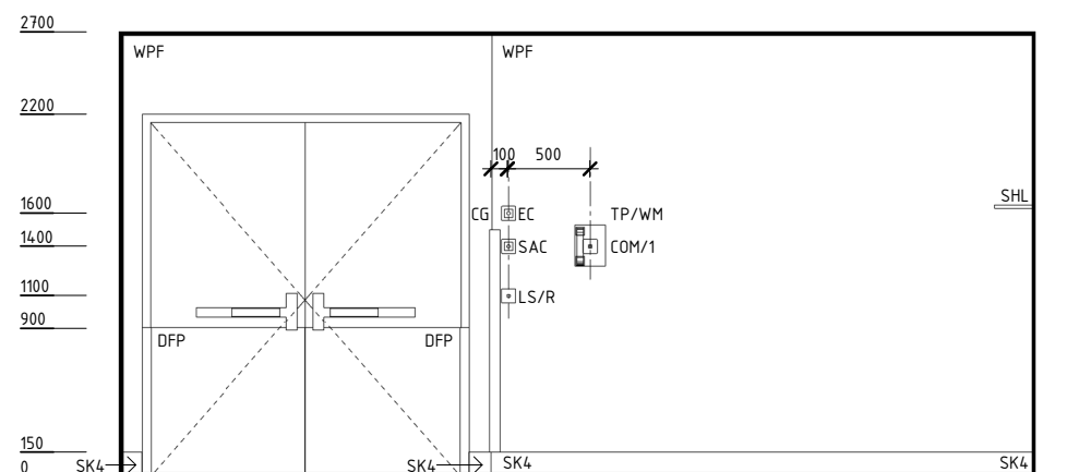
ELEVATION 4
