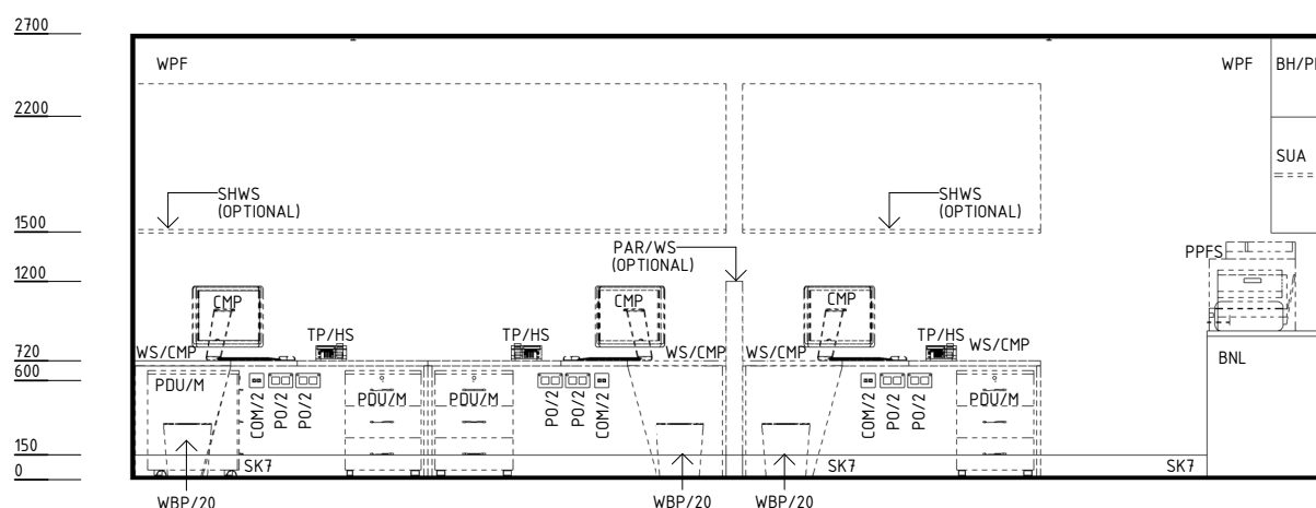
ELEVATION 2
