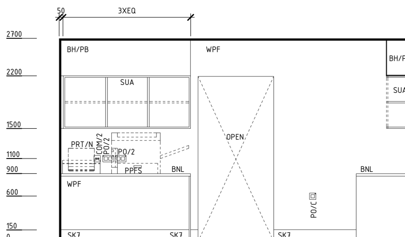
ELEVATION 3
