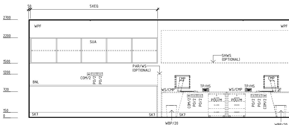
ELEVATION 4
