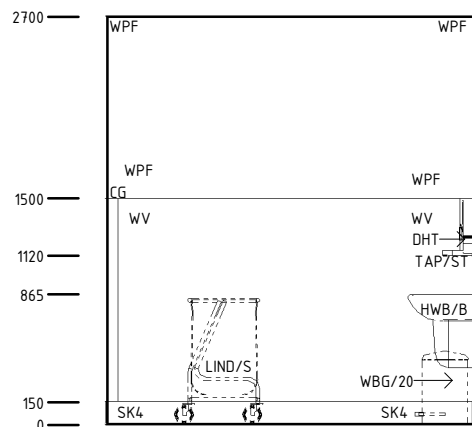
ELEVATION 1
