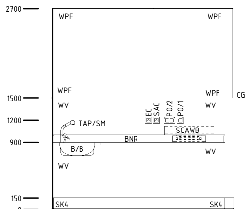
ELEVATION 3
