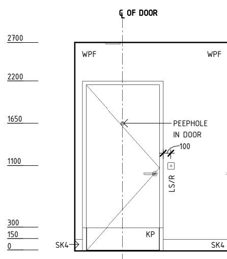
ELEVATION 01
