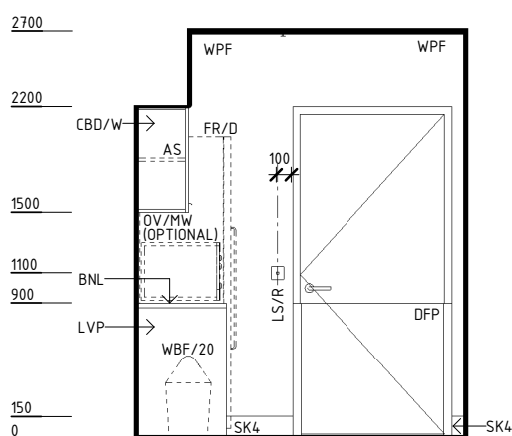
ELEVATION 3
