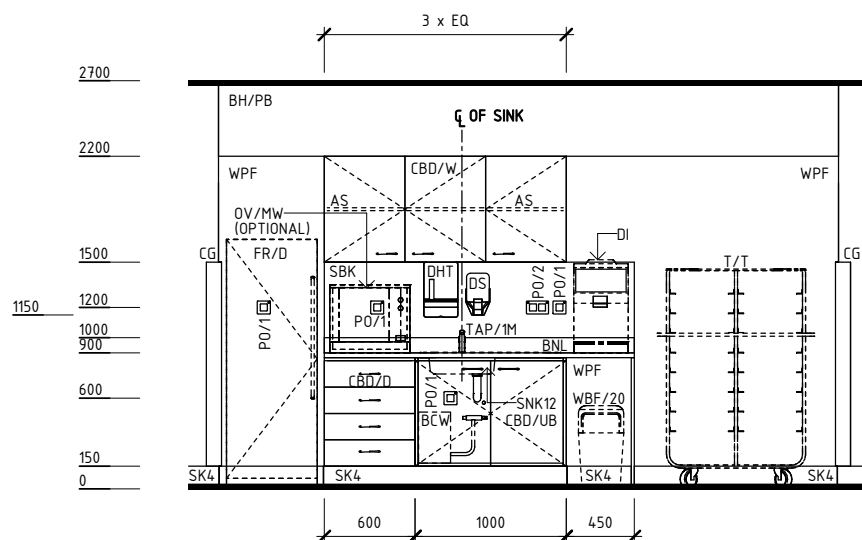
ELEVATION 2
