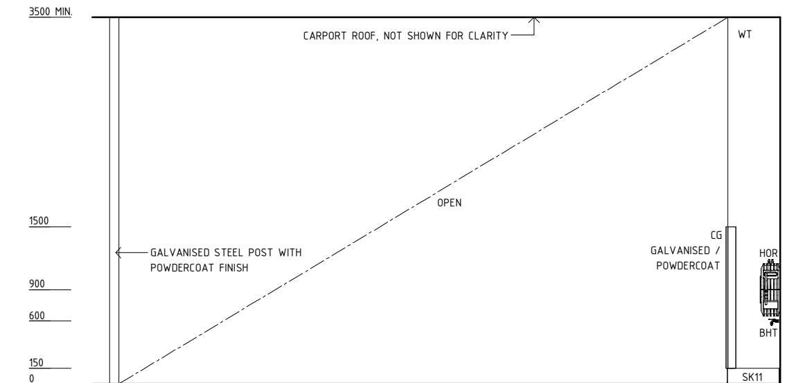
ELEVATION 3
