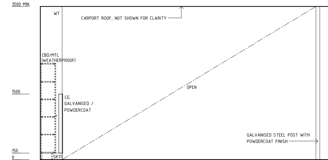
ELEVATION 2
