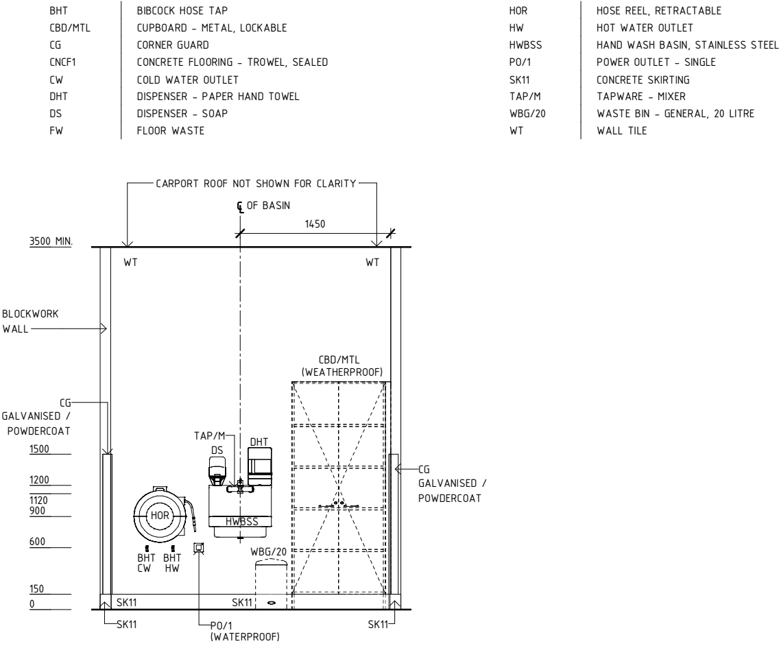
ELEVATION 1
