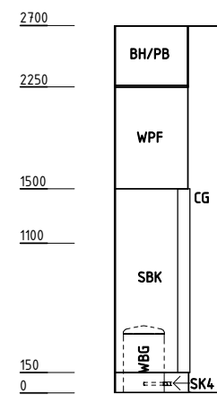
ELEVATION 2
