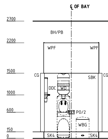
ELEVATION 1
