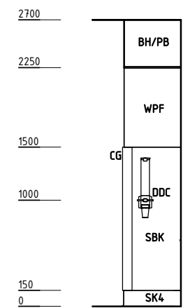
ELEVATION 3
