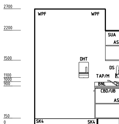
ELEVATION 3
