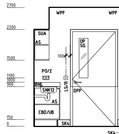
ELEVATION 2
