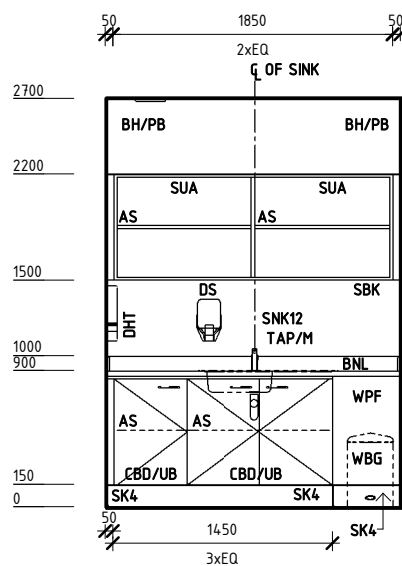
ELEVATION 1
