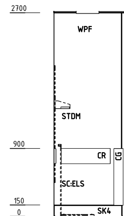
ELEVATION 3
