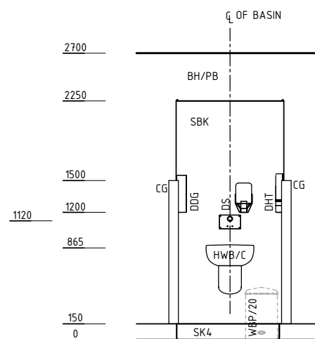
ELEVATION 1
