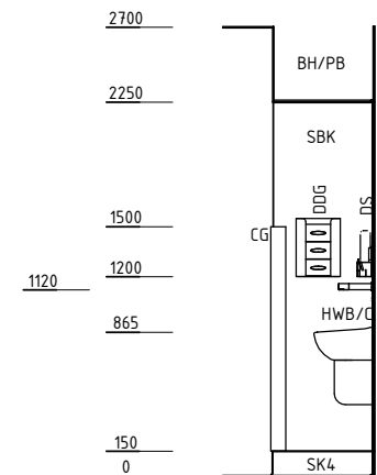
ELEVATION 3
