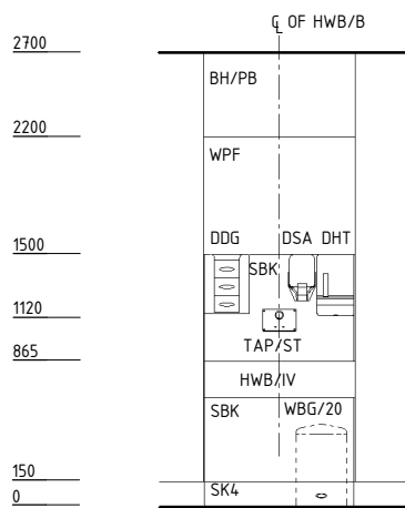
ELEVATION 1
