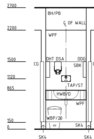
ELEVATION 1
