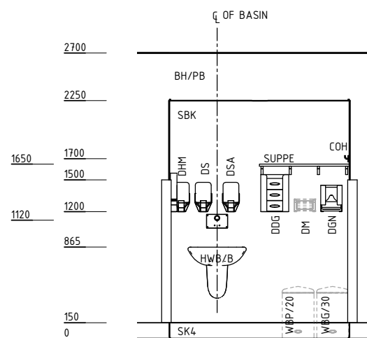
ELEVATION 1
