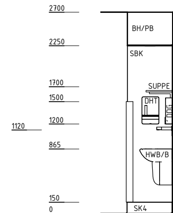
ELEVATION 3
