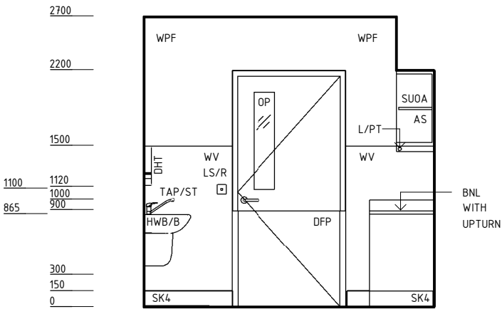
ELEVATION 3
