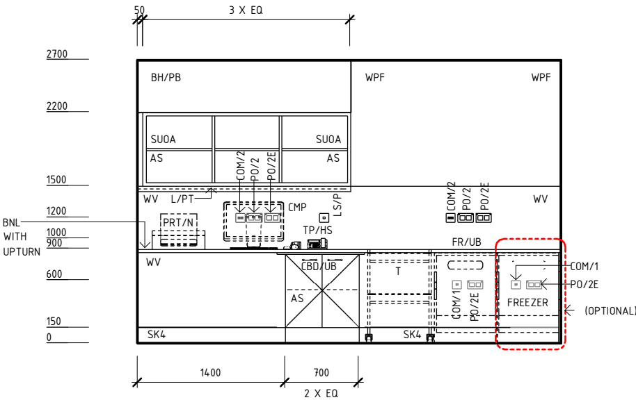
ELEVATION 4
