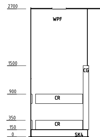
ELEVATION 3
