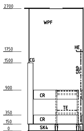
ELEVATION 1
