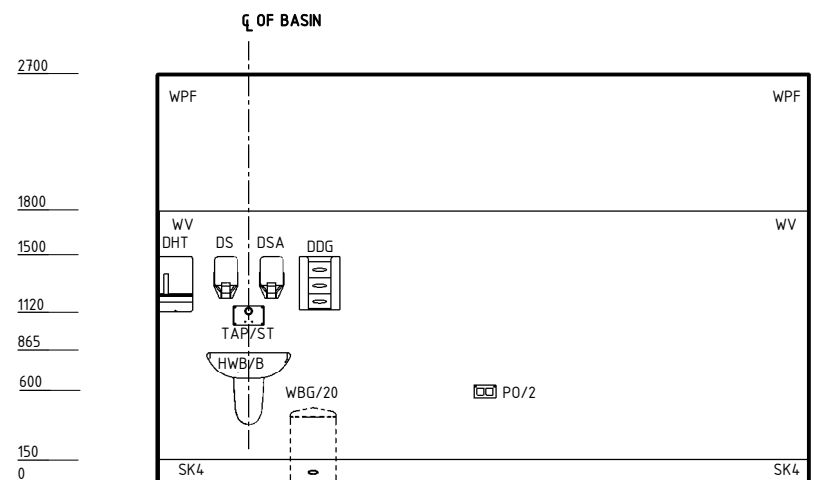
ELEVATION 2
