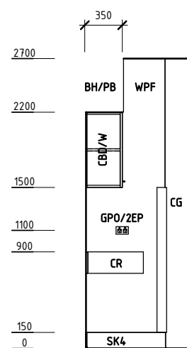
ELEVATION 2
