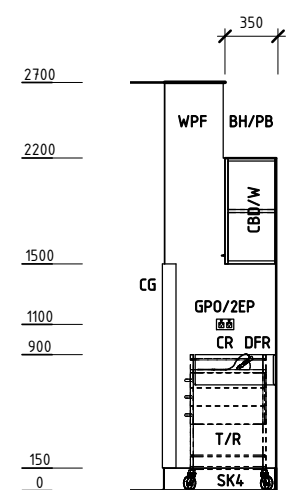
ELEVATION 3
