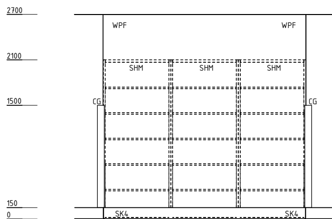
ELEVATION 1
