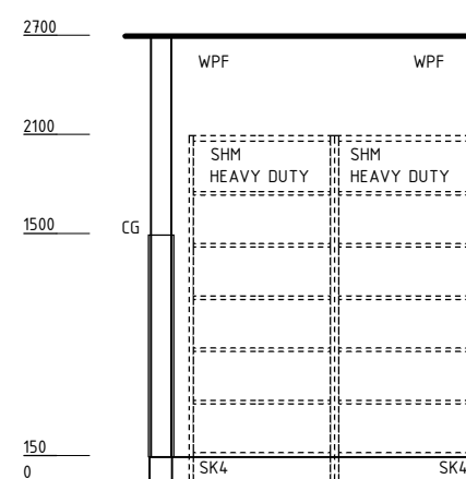
ELEVATION 4
