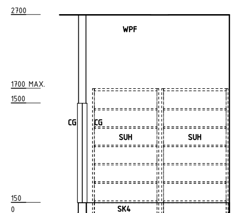
ELEVATION 4
