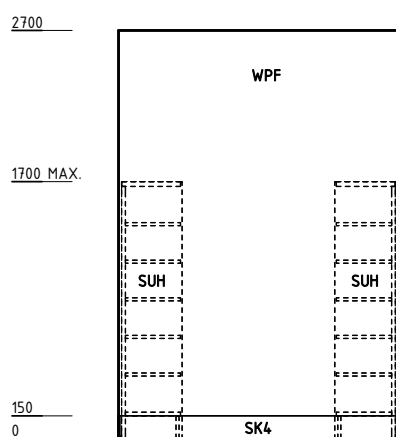
ELEVATION 1
