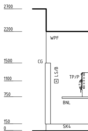
ELEVATION 1
