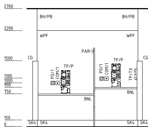
ELEVATION 2
