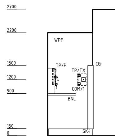
ELEVATION 3
