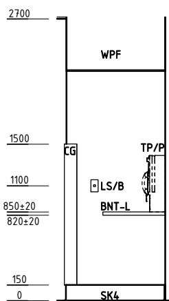
ELEVATION 1
