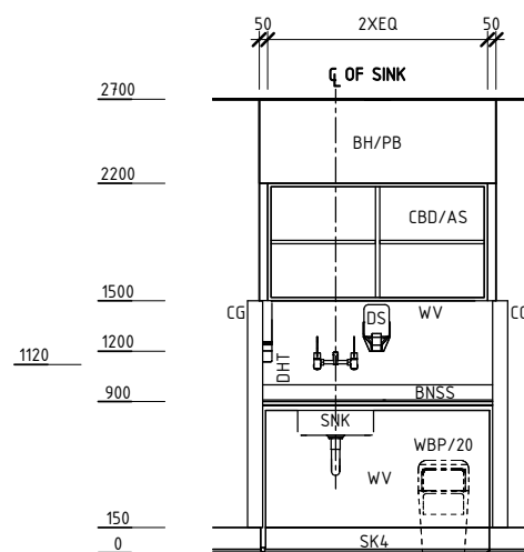
ELEVATION 1
