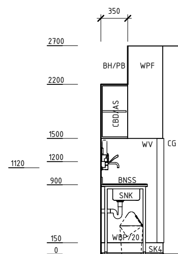
ELEVATION 2
