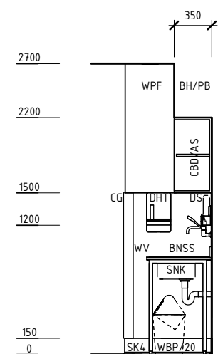
ELEVATION 3
