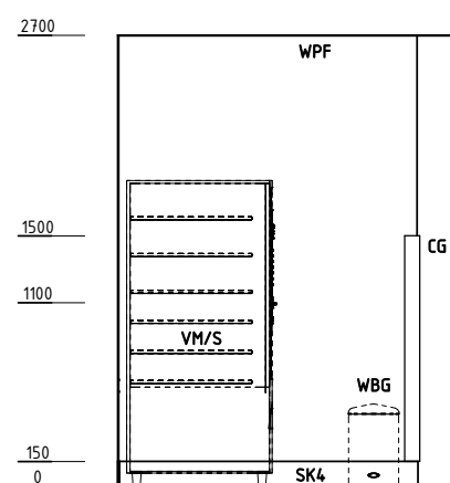
ELEVATION 2
