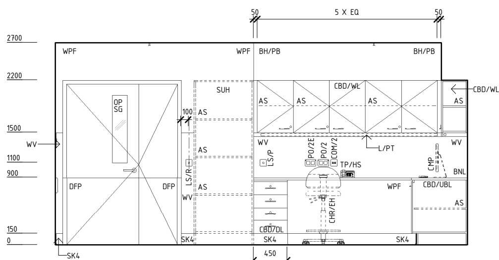
ELEVATION 3
