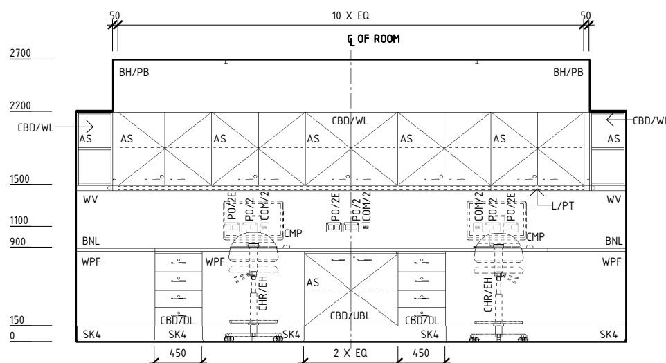
ELEVATION 4
