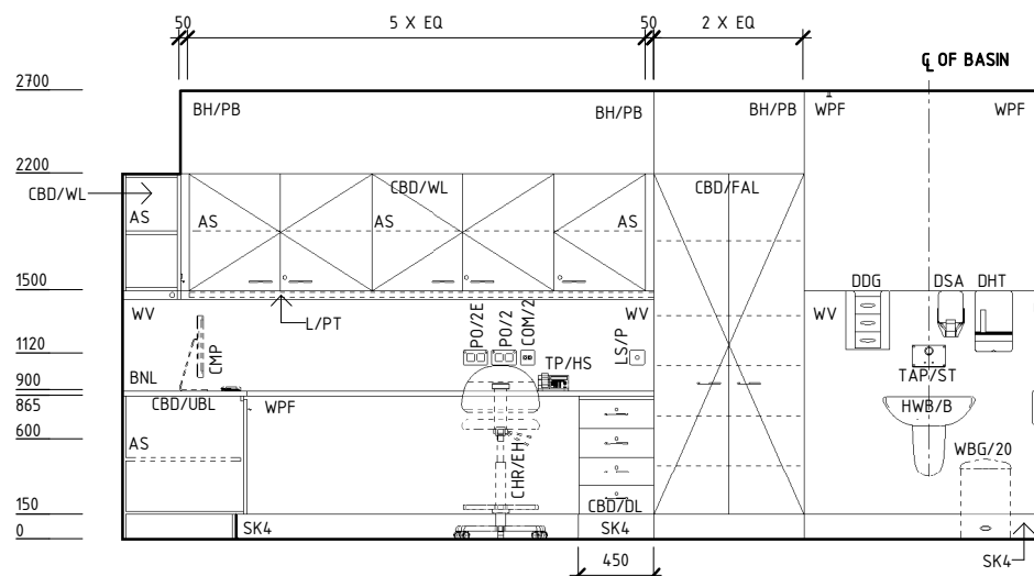
ELEVATION 1
