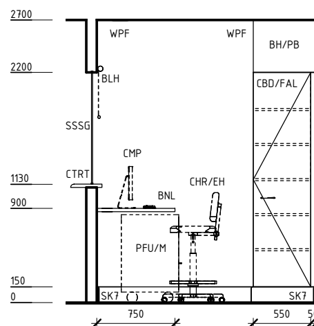
ELEVATION 2
