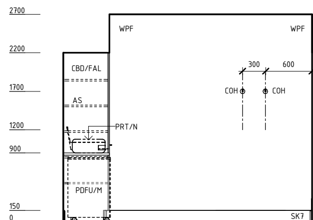
ELEVATION 4
