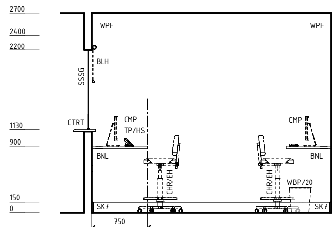
ELEVATION 2
