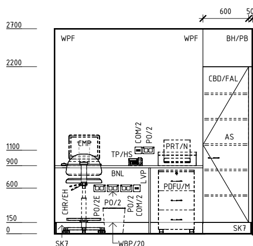
ELEVATION 3
