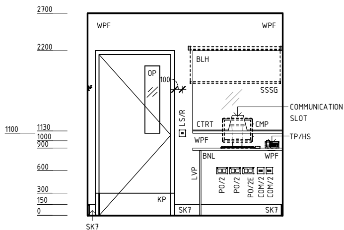
ELEVATION 1
