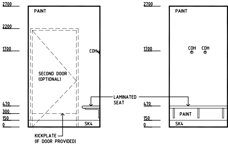
ELEVATION 1
