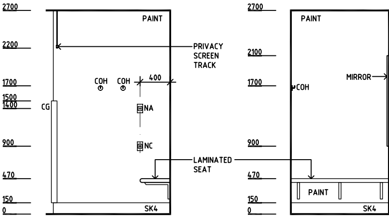
ELEVATION 1
