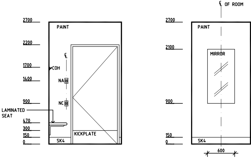
ELEVATION 3
