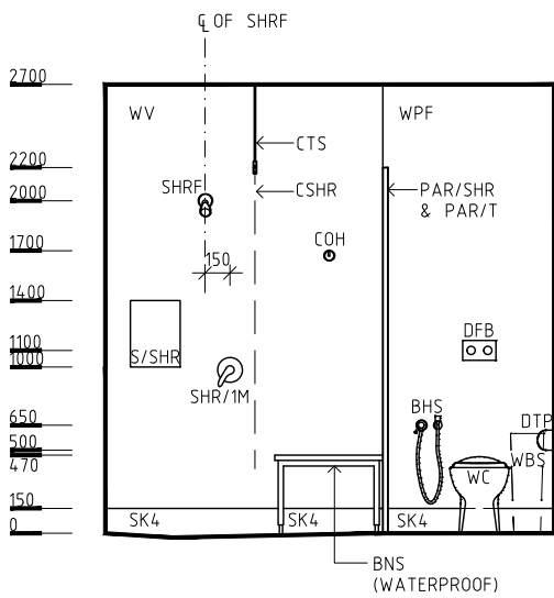
ELEVATION 1
