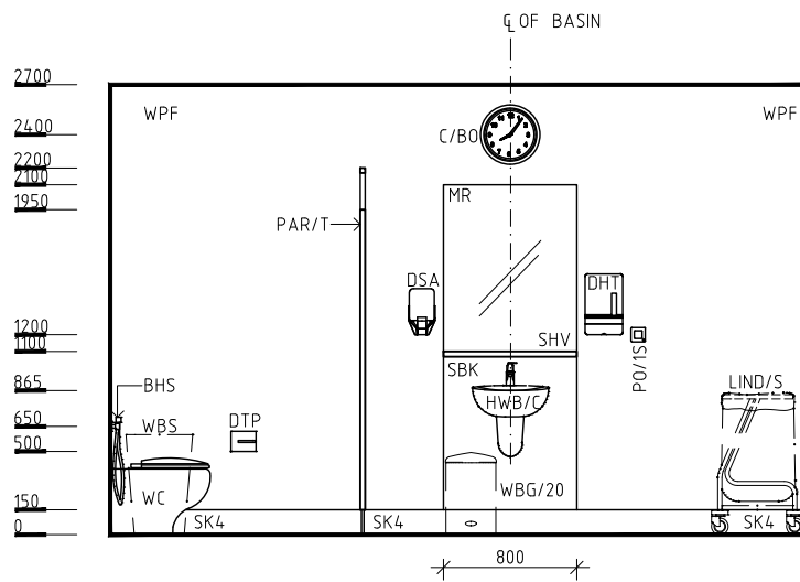
ELEVATION 2
