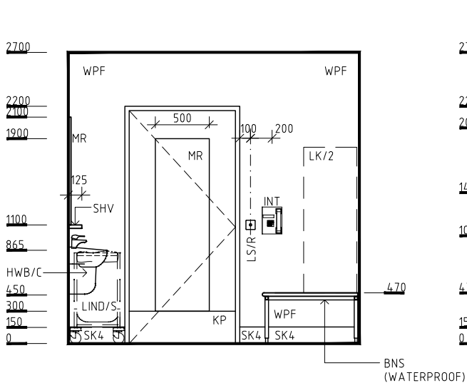
ELEVATION 3
