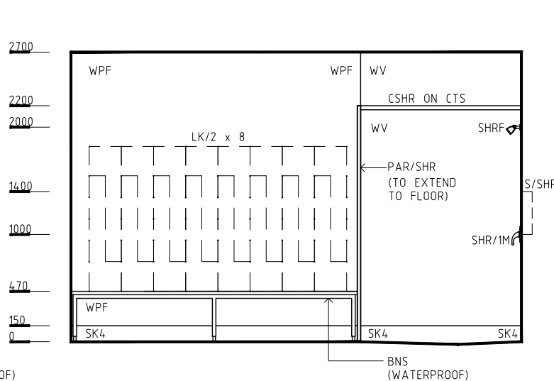
ELEVATION 4
