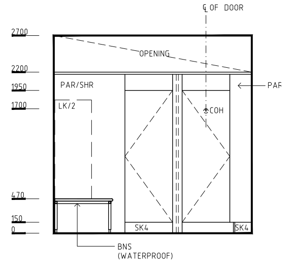
ELEVATION 5
