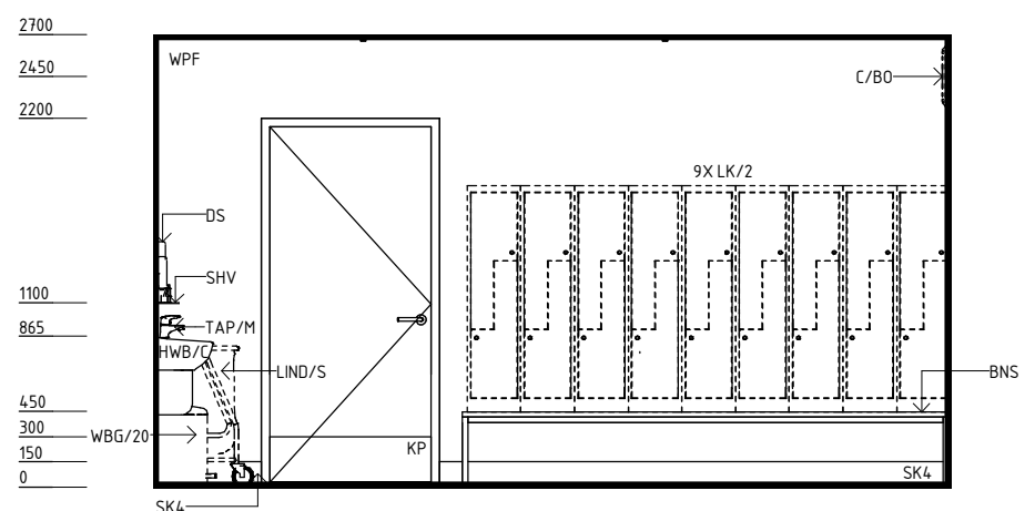
ELEVATION 2
