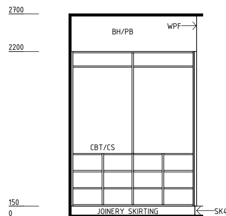
ELEVATION 6
