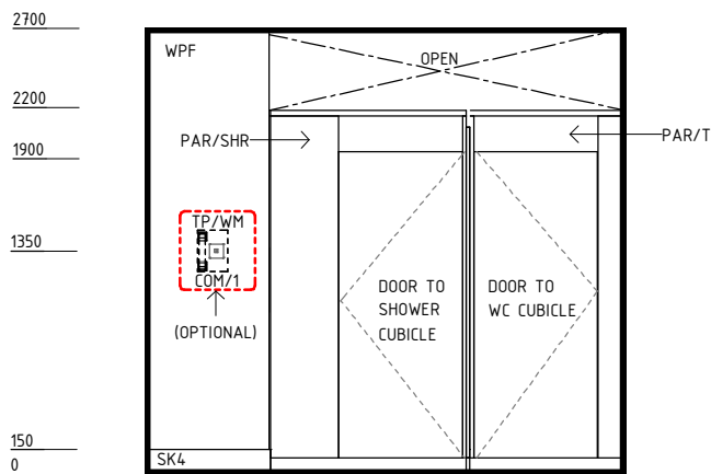
ELEVATION 5
