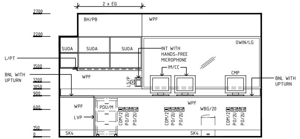
ELEVATION 2
