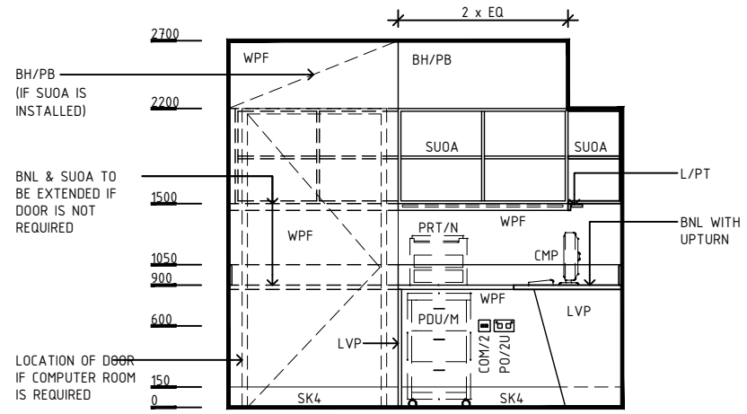
ELEVATION 1
