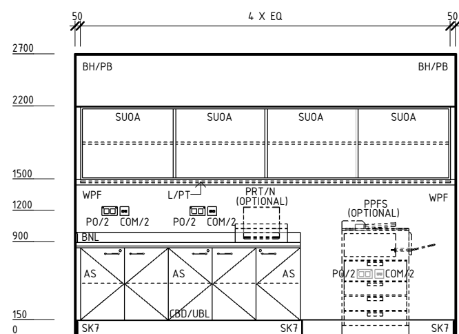
ELEVATION 4
