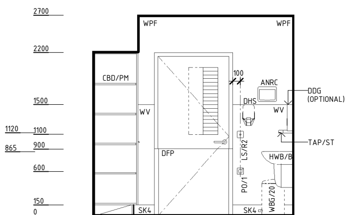
ELEVATION 3
