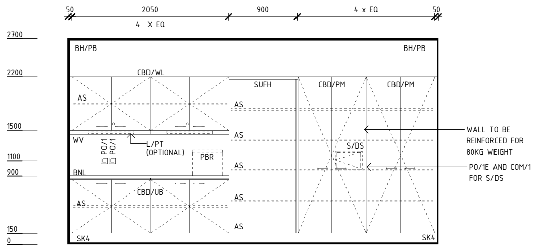
ELEVATION 2
