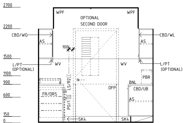
ELEVATION 1
