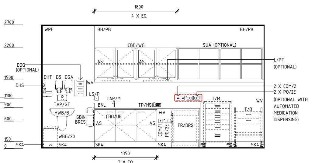
ELEVATION 4
