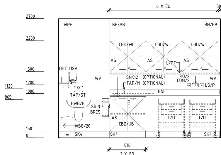
ELEVATION 4
