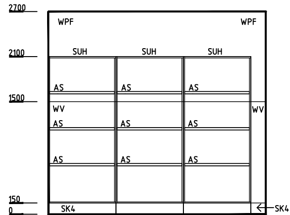
ELEVATION 2
