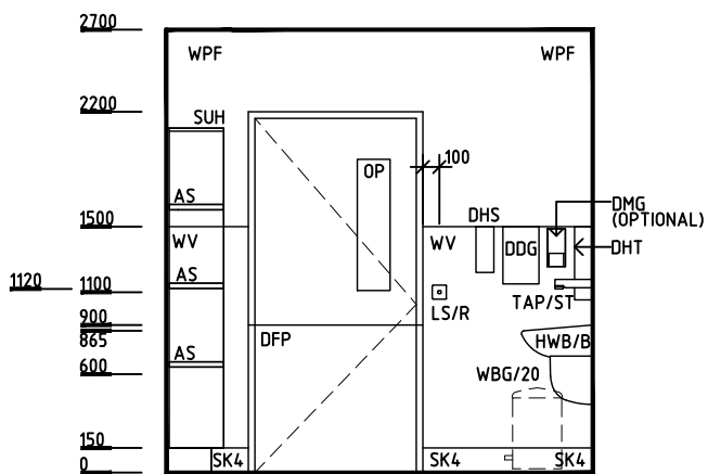
ELEVATION 3
