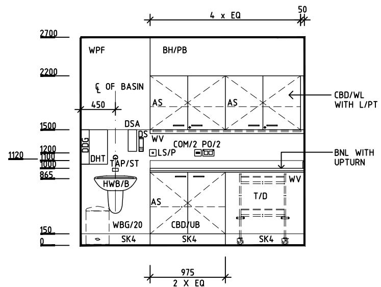
ELEVATION 4
