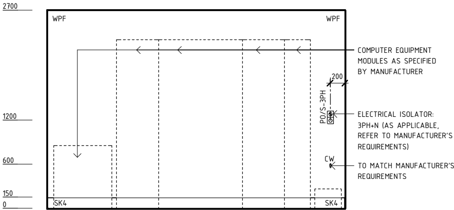
ELEVATION 1
